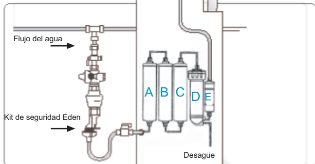
A: Prefiltro B: Filtro de Carbón C-D: Membrana de Osmosis inversa E: Filtro antibacterias
